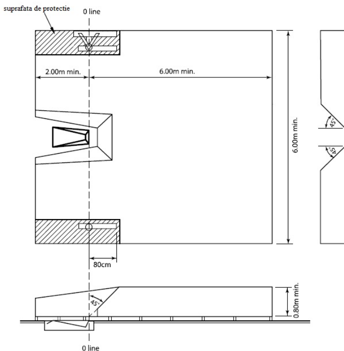
Figura (c) TR28 - Zona de aterizare a săriturii cu prăjină (vederi de sus și laterale)
