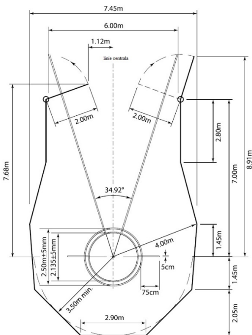
Figura (a) TR37 - Cușcă pentru aruncarea ciocanului și a discului cu cercuri concentrice (configurația pentru aruncarea ciocanului pentru aruncătorul dreptaci cu dimensiunile cuștii față de plasă)
