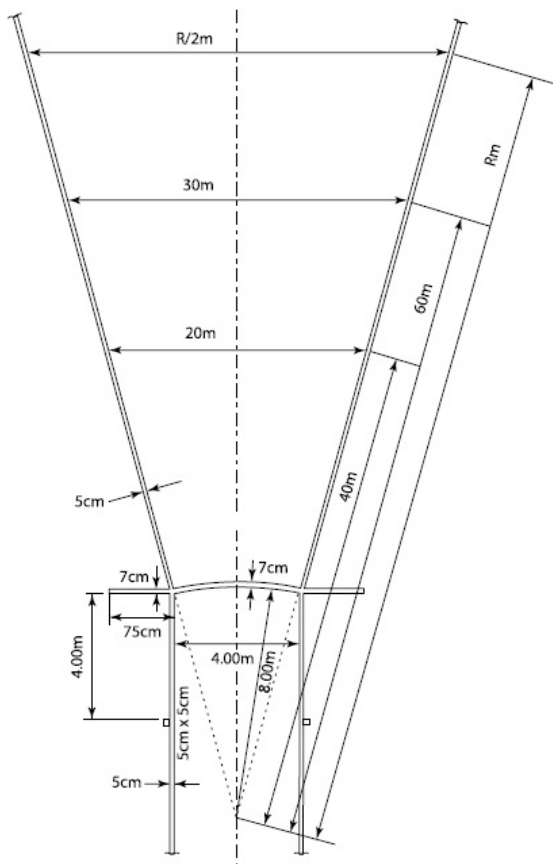
Figura (e) TR32 - Pistă de elan a suliței și sectorul de aterizare (nu este la scară)
