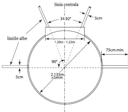
Figura (a) TR32 - Dispunerea cercului de aruncare a greutatei
