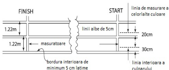
Figura TR14 - Măsurătorile pistei (vedere în teren)
